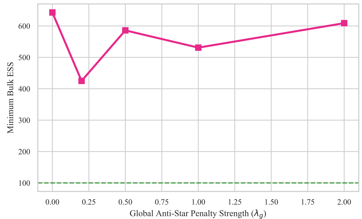
(D) Phase 3 Sample Information Capacity
